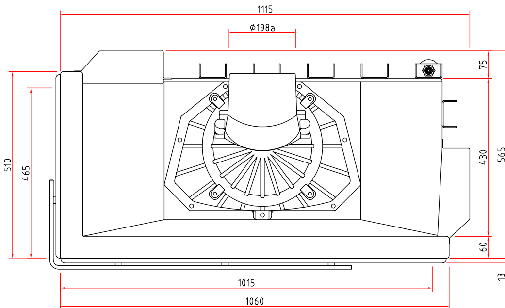
Draufsicht M 1:10
