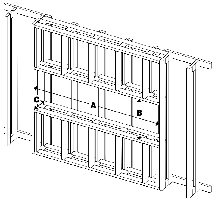
Abbildung 10 Frontinstallation
